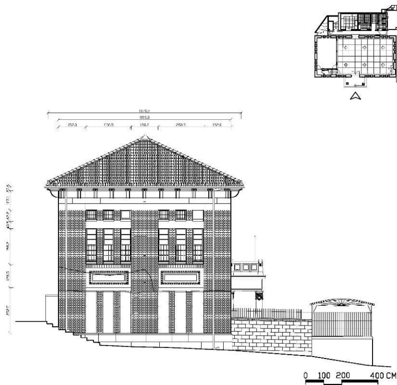
右側立面現況圖
