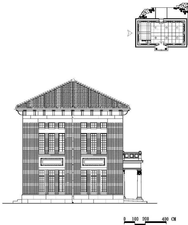
右側立面復原圖
