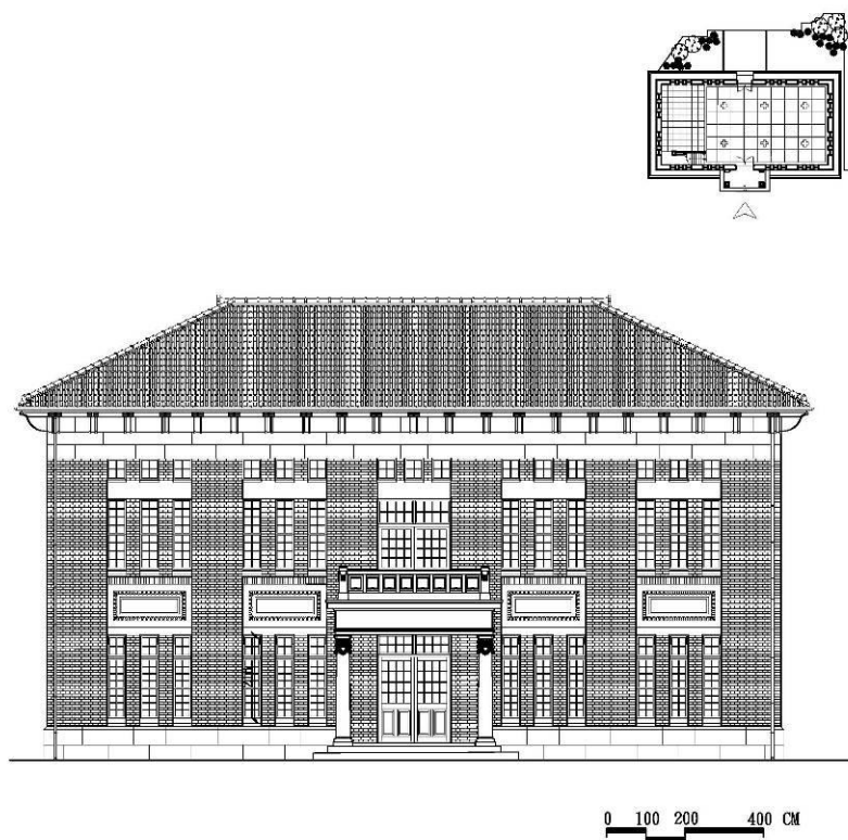
正立面復原圖
