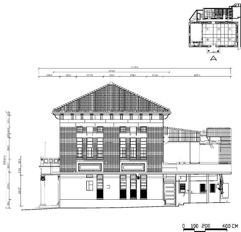
左側立面現況圖
