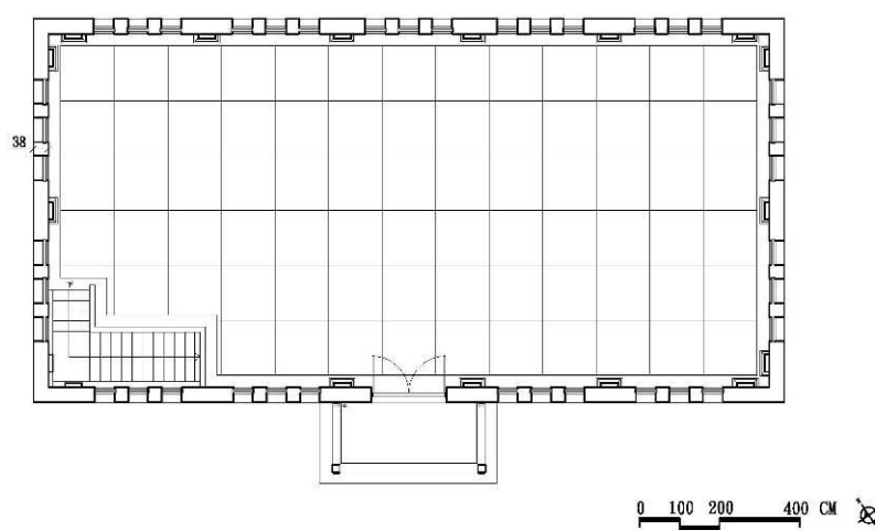
二層平面復原圖
