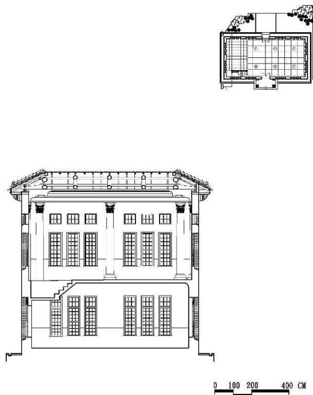
D-D 剖面復原圖
