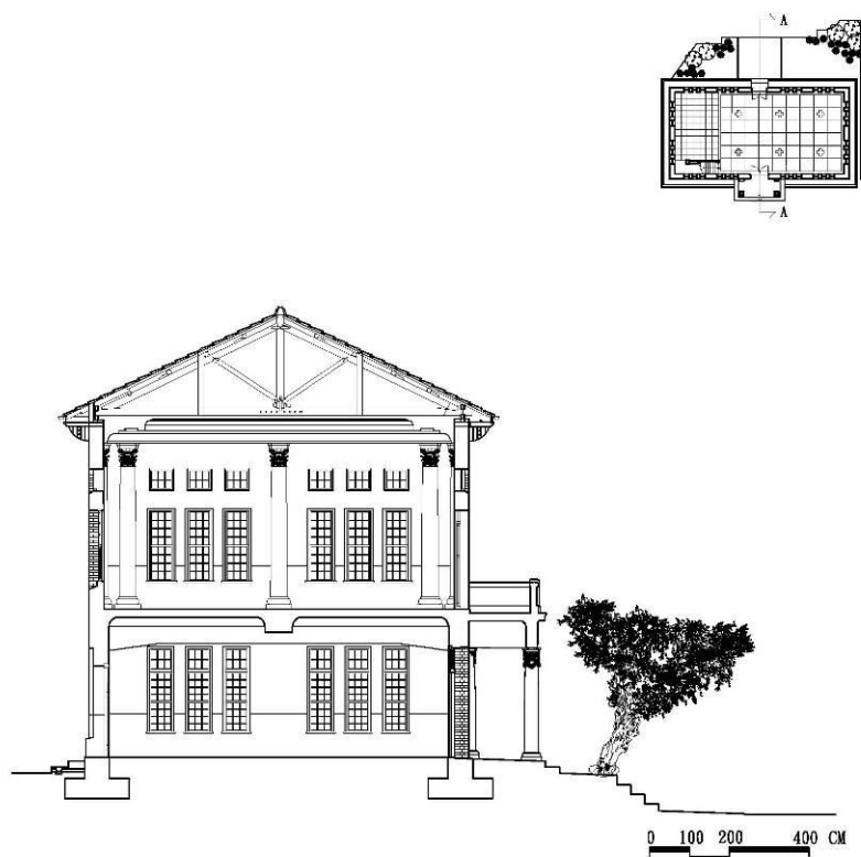
A-A 剖面復原圖
