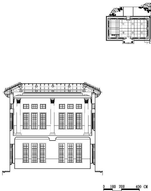
C-C 剖面復原圖
