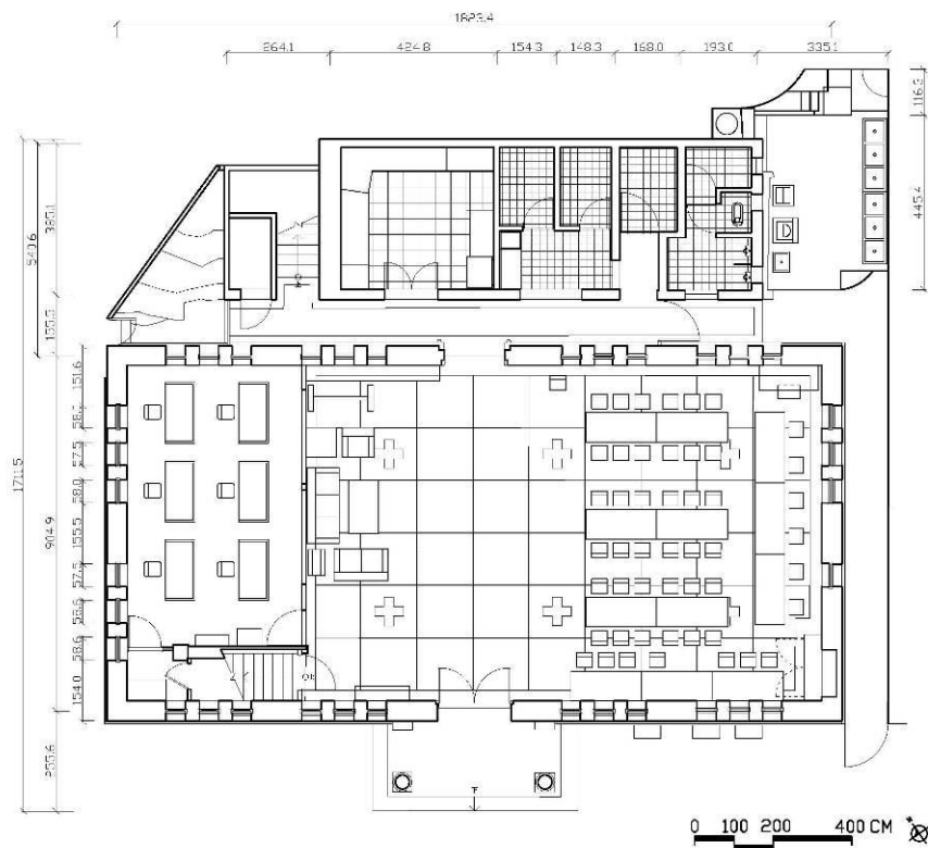
一層平面現況圖
