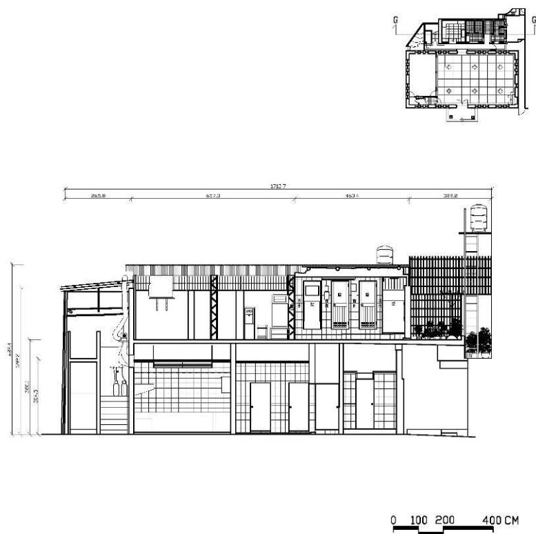
G-G 剖面現況圖
