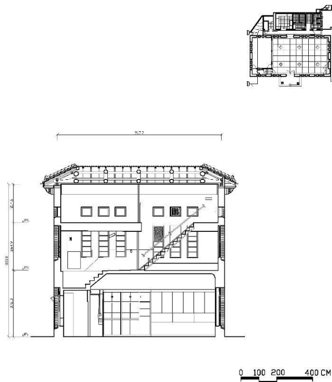
D-D 剖面現況圖
