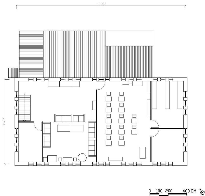
增建夾層平面現況圖
