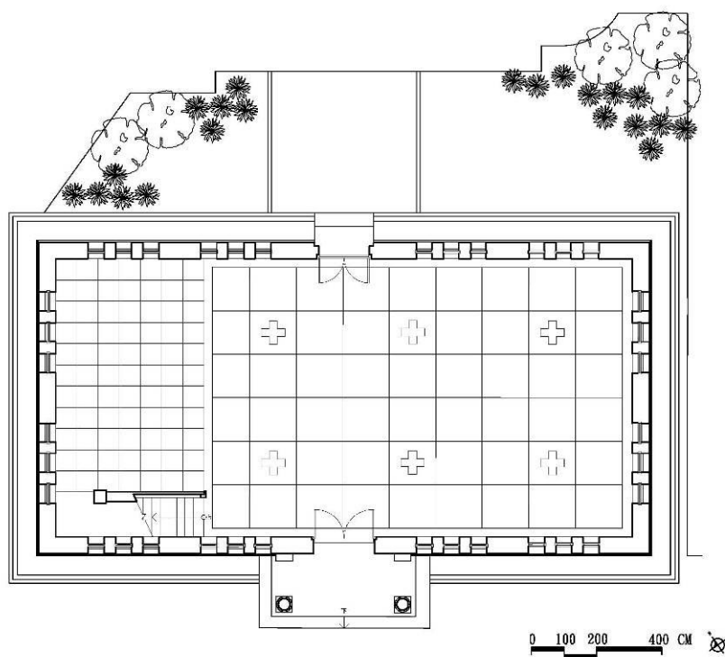
一層平面復原圖
