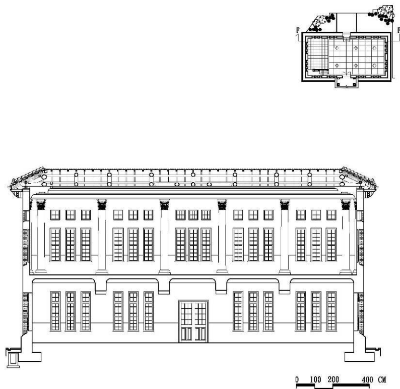
F-F 剖面復原圖
