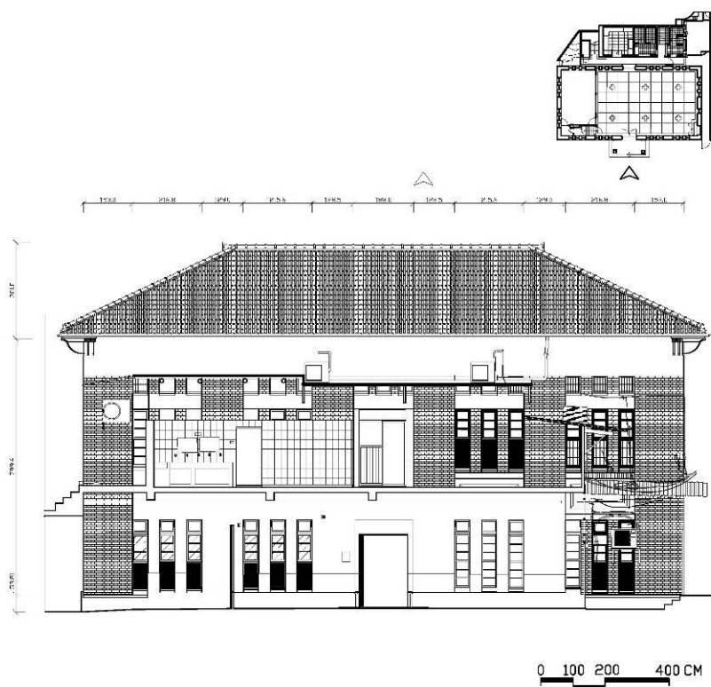
背立面現況圖
