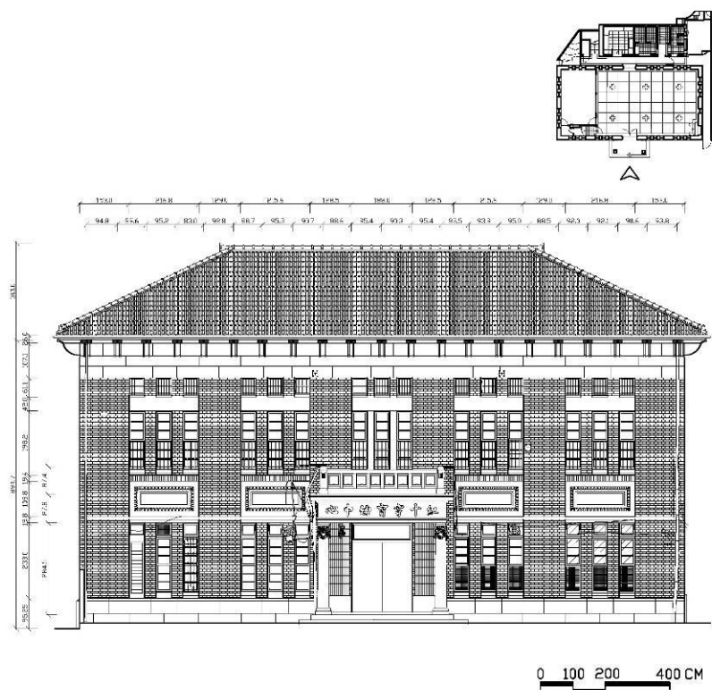
正立面現況圖
