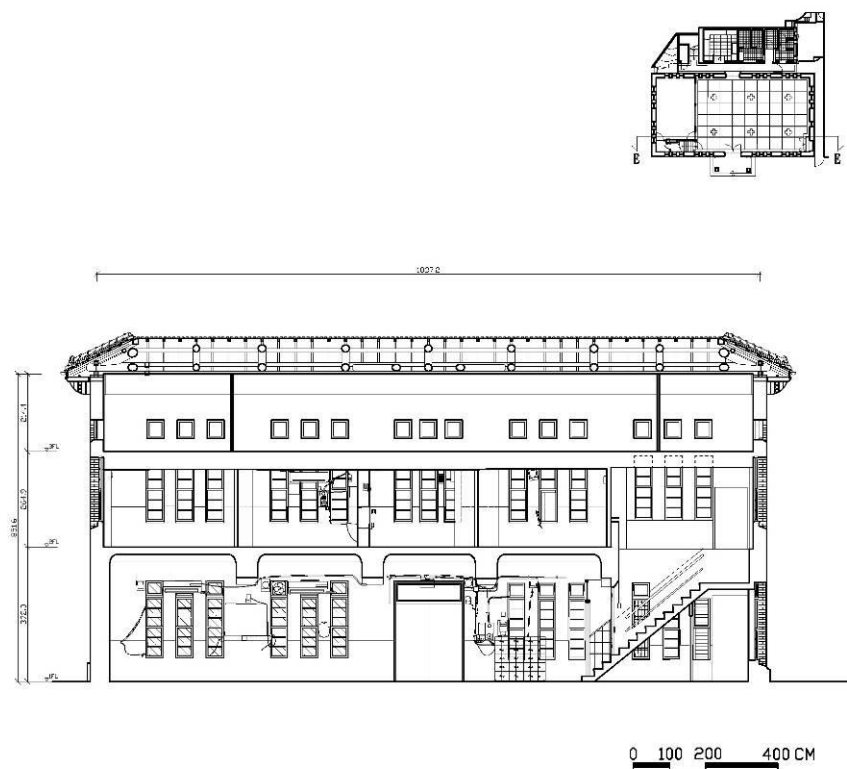
E-E 剖面現況圖
