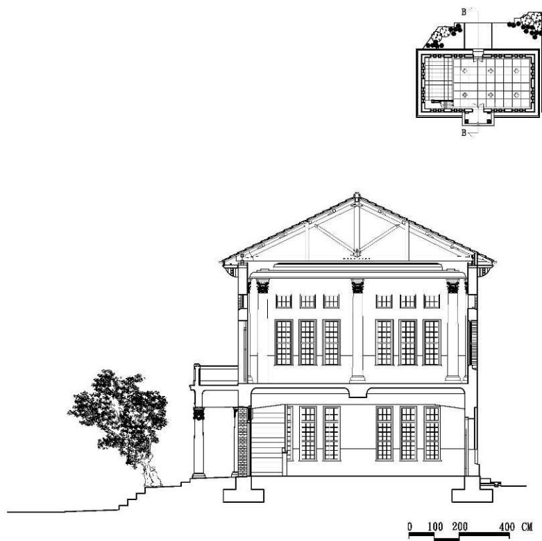
B-B 剖面復原圖
