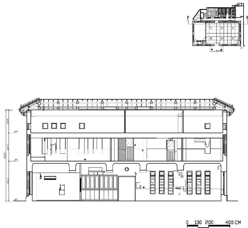
F-F 剖面現況圖
