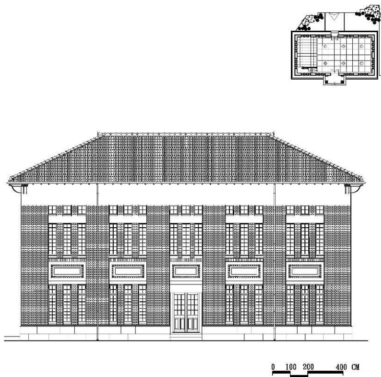
背立面復原圖
