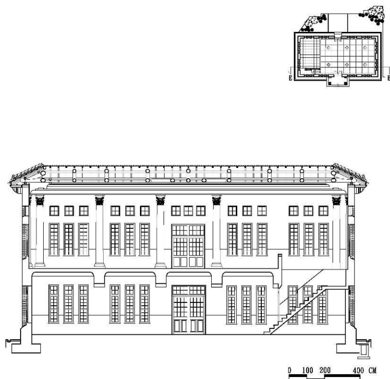
E-E 剖面復原圖
