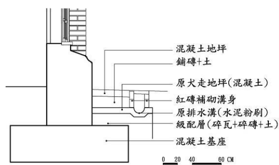
圖 2-8 原犬走地坪及排水溝圖
